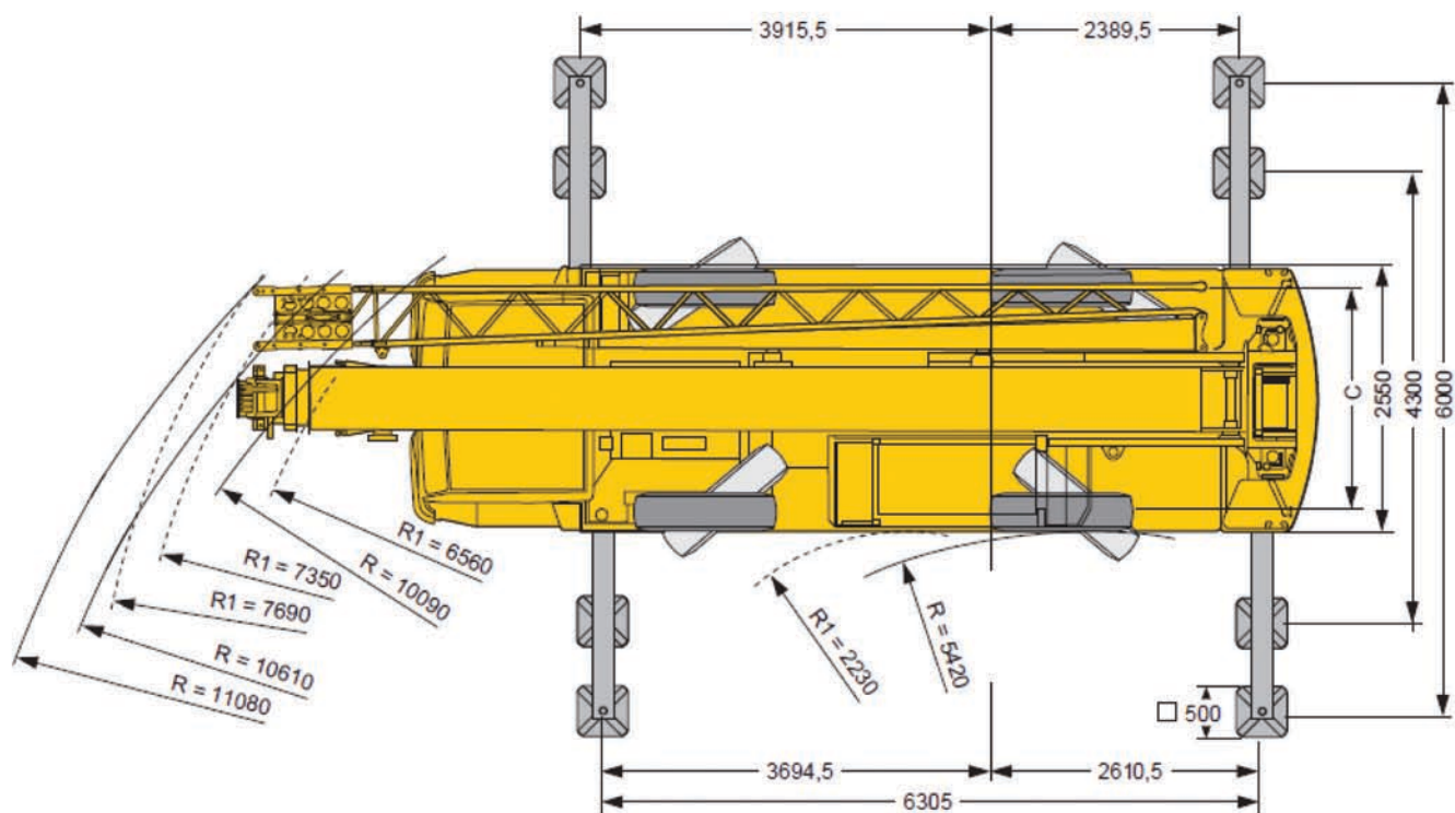
Wymiary · Maße · Dimensions
